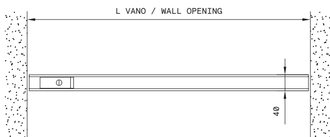
MECCANISMO LATERALE / LATERAL MECHANISM
