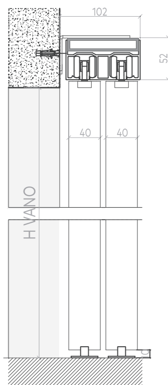
BINARIO DOPPIO DOUBLE WALL TRACK
