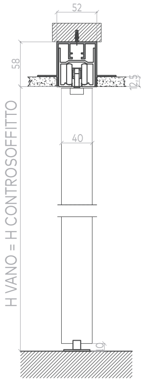
BINARIO SINGOLO CARTONGESSO CONCEALED SINGLE TRACK
