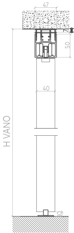
BINARIO SINGOLO SINGLE CEILING TRACK
