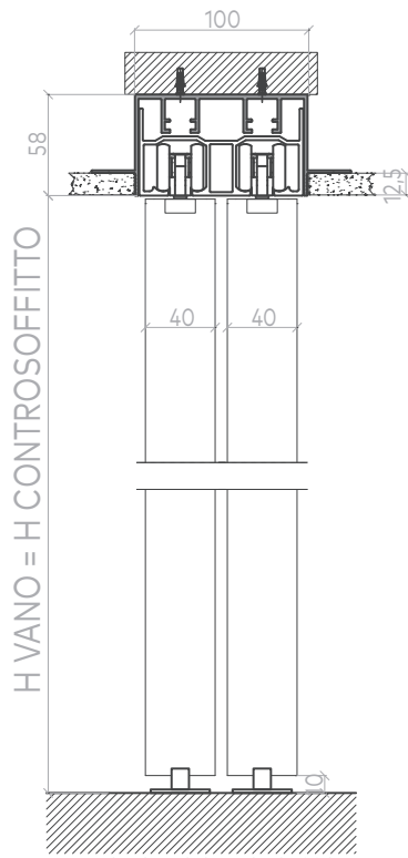
BINARIO DOPPIO CARTONGESSO CONCEALED DOUBLE TRACK
