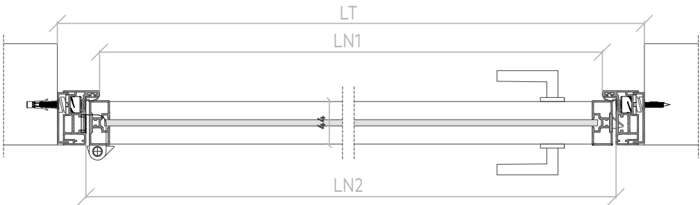
Sezione orizzontale Horizontal section
