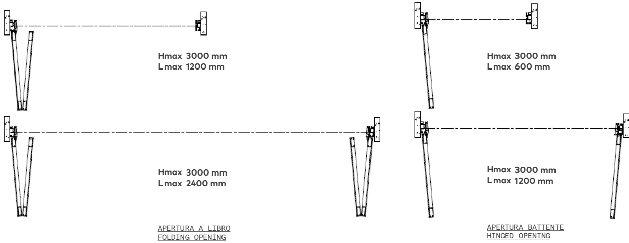
Esempi di composizione Composition examples
