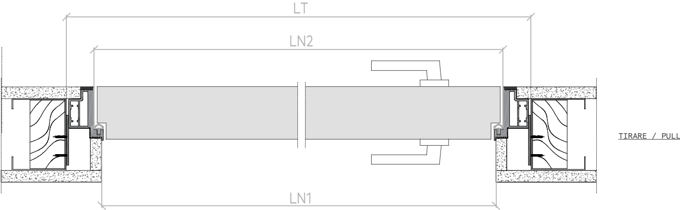
Sezione verticale Vertical section
