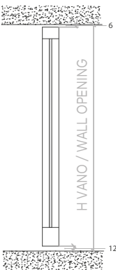
Sezione verticale Vertical section
