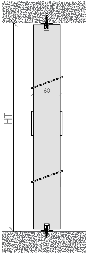
Sezione verticale Vertical section
