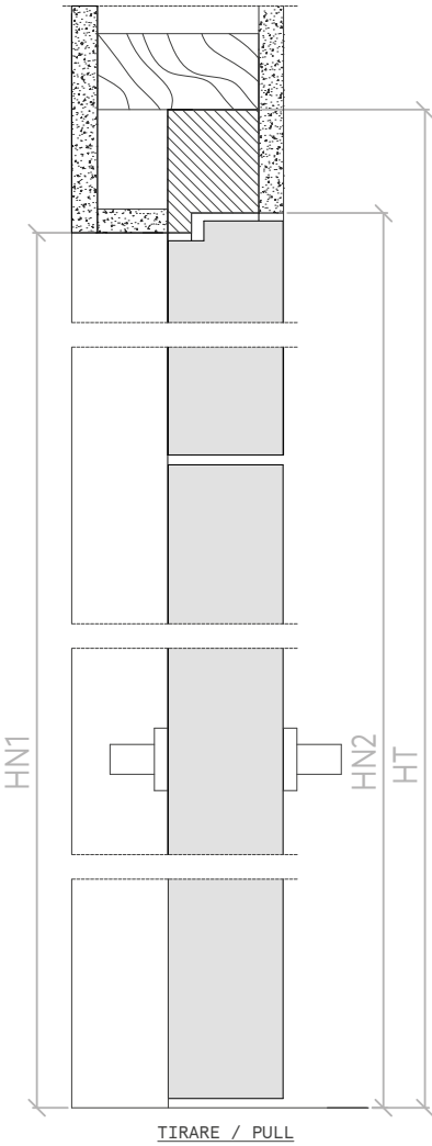
Sezione verticale Vertical section
