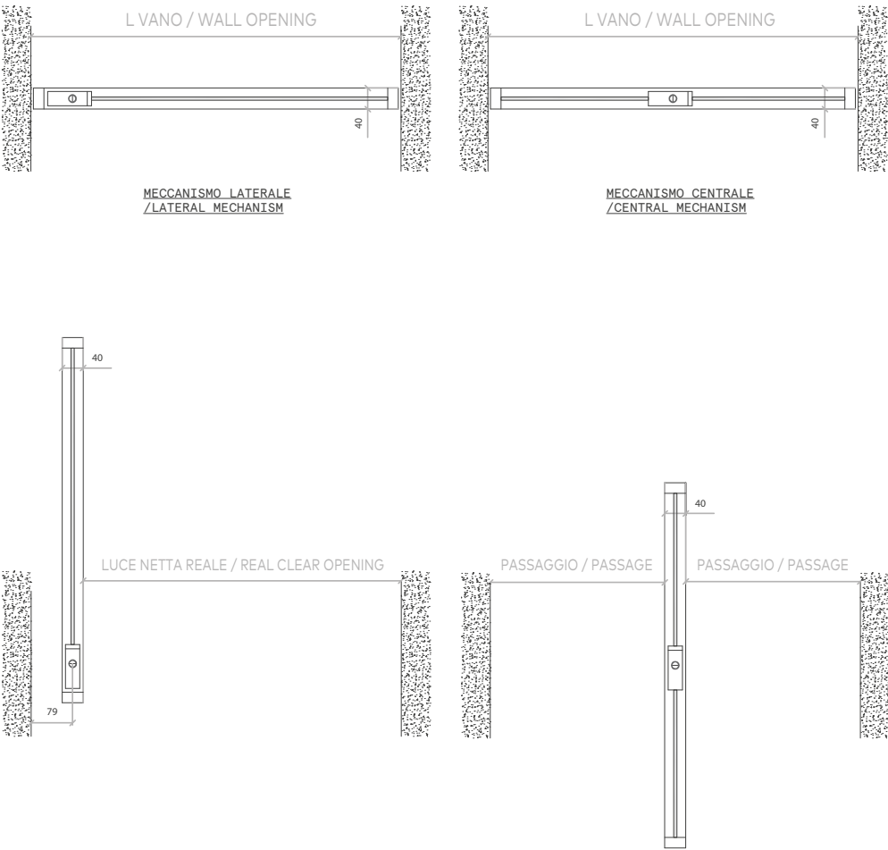
Sezione orizzontale Horizontal section
