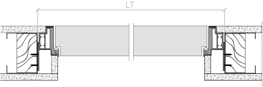
Dettaglio telaio V0 ARCO Detail V0 ARCH frame
