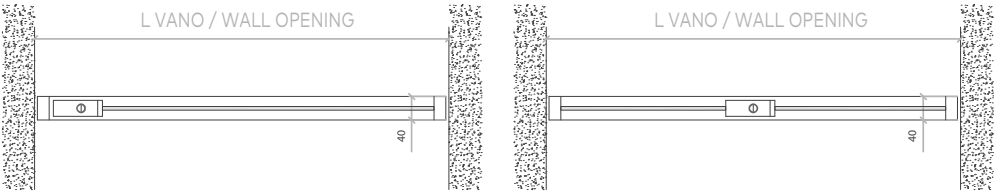
MECCANISMO LATERALE / LATERAL MECHANISM
