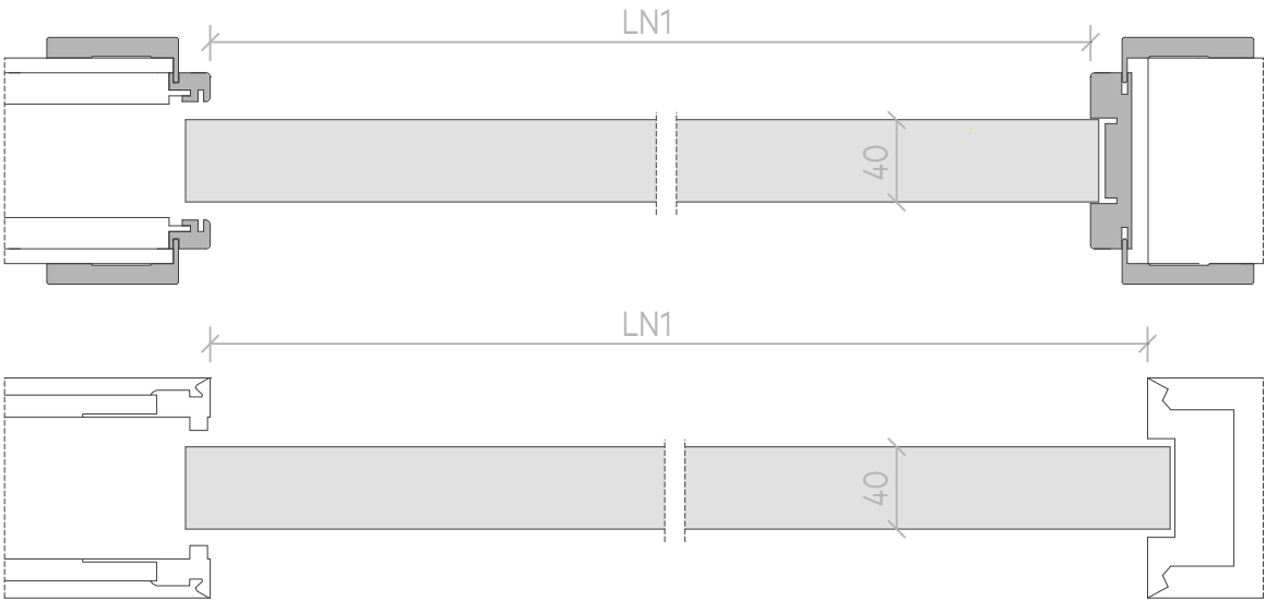
Sezione orizzontale Horizontal section
