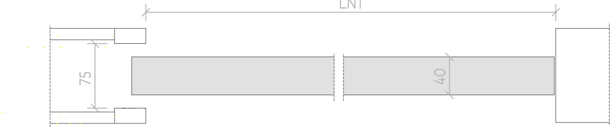
Sezione orizzontale Horizontal section
