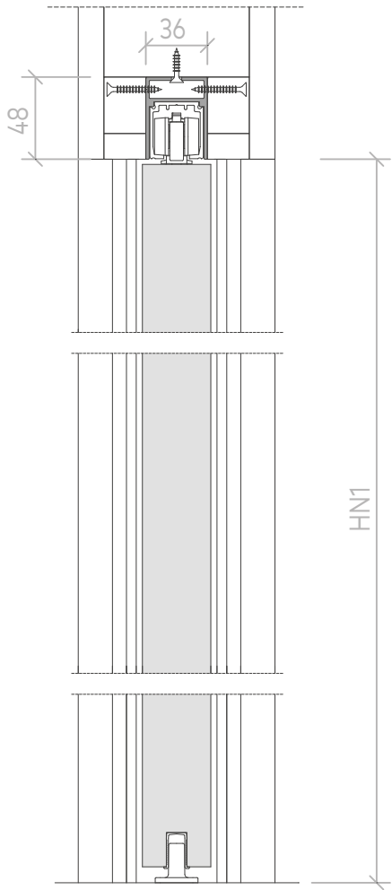
Sezione verticale Vertical section
