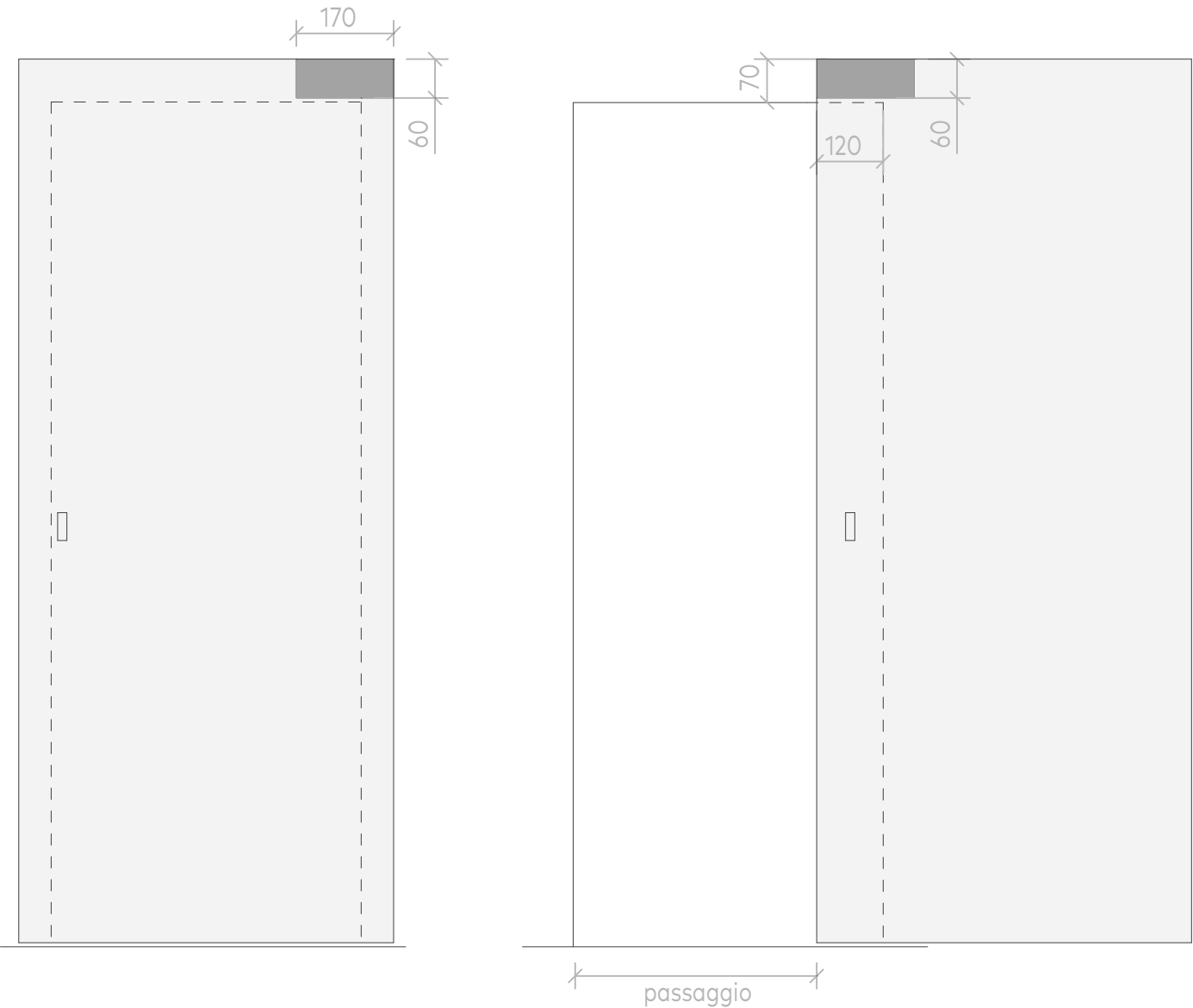
Posizione meccanismo Hardware position
